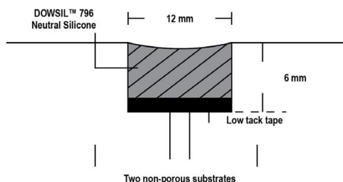
Obr. 2: Plytký spoj
