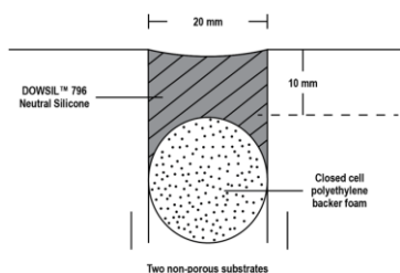
Obr. 1: Hlboký spoj
