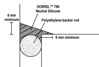
Obr. 3: Rohový spoj
